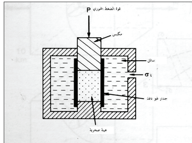
الشكل ١ :- رسم مبسط لضاغطة ثلاثية المحاور (M.Mattauer, 1980)
