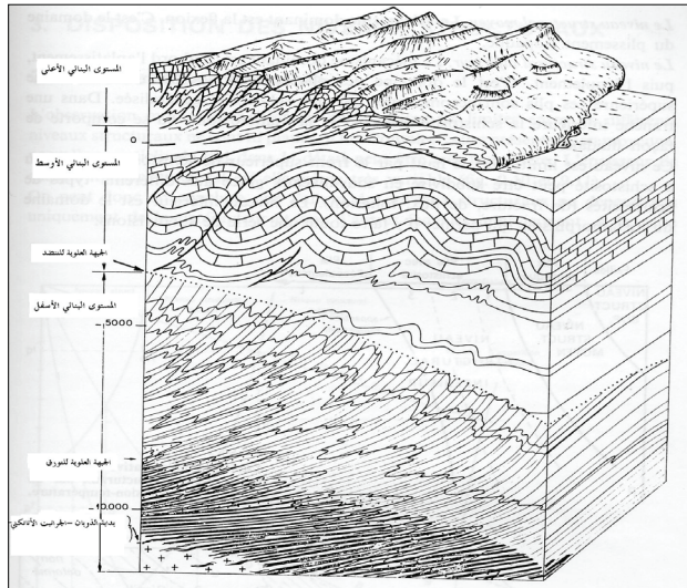
الشكل 7:- مقطع نظري لجزء من القشرة الأرضية بين المستويات البنائية الرئيسية ونوعية البنيات المقابلة لها (M.Mattauer, 1980)
