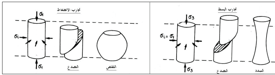
الشكل ٢ :- تمثيل لنتائج تشوه عينة صخرية خلال تجرب الانضغاط وتجارب البسط (M.Mattauer, 1980)
