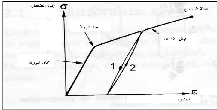
الشكل 4 :- منحنى العلاقة بين قوة الضغط والتشوه في حالة جسم مرن-لدن (M.Mattauer,1980)
